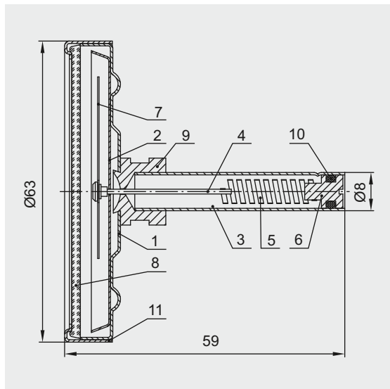
Термометр биметаллический PROFACTOR® PF SG 868:
