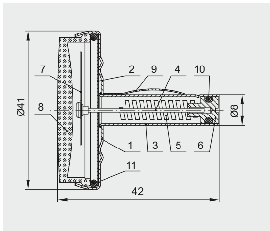
Термометр биметаллический PROFACTOR® PF SG 866:
